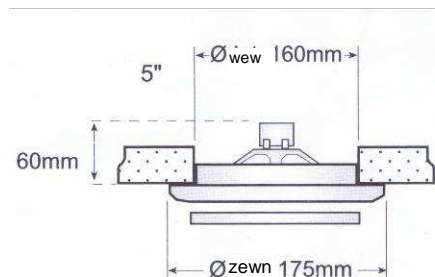
Rys. 2. Sposób montażu dla typu 05072-39
