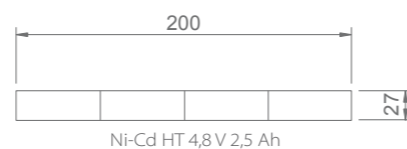
Ni-Cd HT 4,8 V 2,5 Ah
