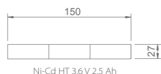
Ni-Cd HT 3,6 V 2,5 Ah
