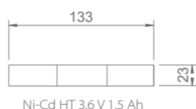
Ni-Cd HT 3,6 V 1,5 Ah
