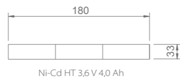
Ni-Cd HT 3,6 V 4,0 Ah
