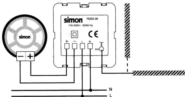
SCHEMAT PODŁĄCZENIA GŁOŚNIKÓW
