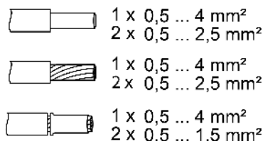
Rysunek 4: Przekrój przewodów do zacisków
