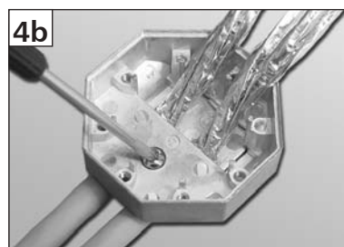
Anschlussdose 2fach wall outlet 2-gang
