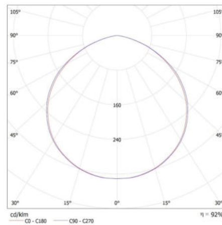
MILED0 (kat 31396) GRUN NV LED-200-B / LDC (Polar) Luminaire: MILED0 (kat 31396) GRUN NV LED-200-B Lamps: 1 x GRUN NV LED-200-B
