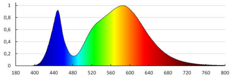
MILED0 (kat 31396) GRUN NV LED-200-B / LDC (Polar) Luminaire: MILED0 (kat 31396) GRUN NV LED-200-B Lamps: 1 x GRUN NV LED-200-B
