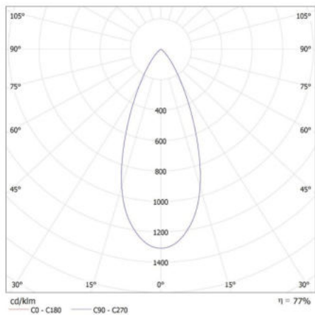
KANLUX S.A. (kat 35658) BTL 38W-930-W 45deg + GRID / LDC (Polar)
