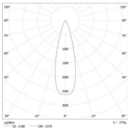
KANLUX S.A. (kat 35658) BTL 38W-930-W 15deg + GRID / LDC (Polar)
