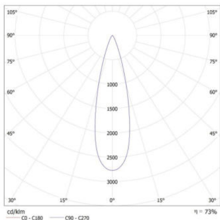
KANLUX S.A. (kat 35659) BTL 38W-930-B 15deg + GRID / LDC (Polar)
