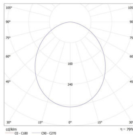
KANLUX S.A. (kat 35677) TIBERI PRO NT20W-940B / LDC (Polar)
