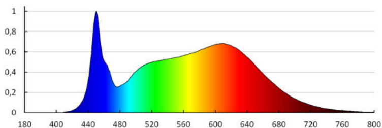
KANLUX S.A. (kat 35677) TIBERI PRO NT20W-940B / LDC (Polar)
