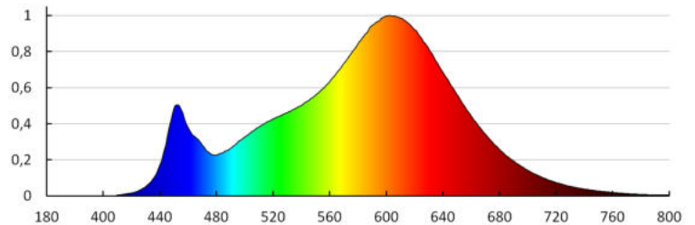
KANLUX S.A. (kat 36461) RIFA LED 17,5W WW / LDC (Polar)
