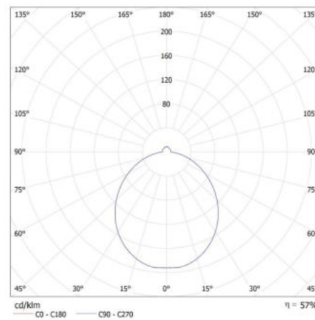
KANLUX S.A. (kat 36461) RIFA LED 17,5W WW / LDC (Polar)
