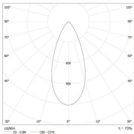
KANLUX S.A. (kat 35661) BTL 38W-940-B 45deg + GRID / LDC (Polar)
