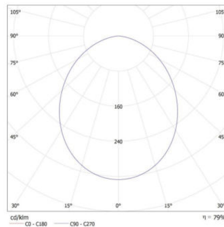
KANLUX S.A. (kat 35676) TIBERI PRO NT20W-940W / LDC (Polar)
