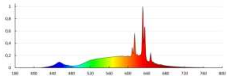
KANLUX S.A. (pat 36682) IQ-LED C35E14 3,4W-WW / Krzywa rozkładu światła (Współczynniki)
