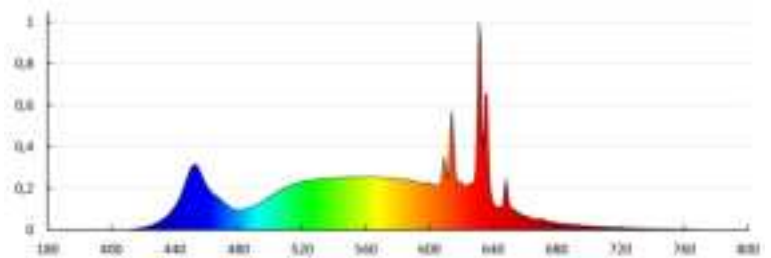
KANLUX S.A. (z siedzibą w Warszawie) IQ-LED G45E14 3,4W-NW - Krzywa mocy światła (względowa)
