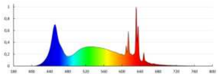
KANLUX S.A. (zad. 36696) IQ-LED G45E14 5,9W-CW / Krzywa mocy światła (względowa)
