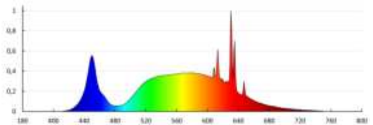
KANLUX S.A. (ser. 37179) BLINGO U24W 4000 60NW / Krzywa mocy światła (Bieganywa)
