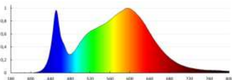
KANLUX S.A. (368 37320) LUMKO LED 17,5W NW / Krzywa mocy światła (Współczynniki)
