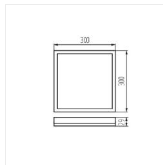
AZPO LED 17,5W-NW-L-B
