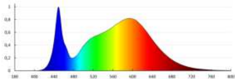
KANLUX S.A. (pat.37303) IPER LED 19W-NW-L-SE / Krzywa mocy światła (długościowe)
