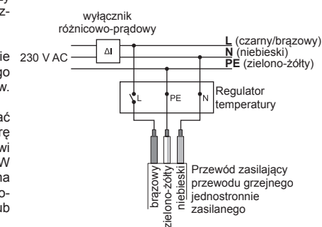
Rys. Schemat podłączenia przewodu grzewczego za pośrednictwem regulatora temperatury do instalacji elektrycznej.
