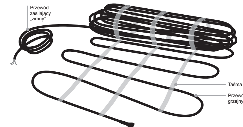
Rys. Mata grzewcza GMPD
