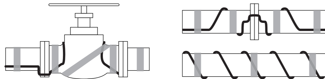
Rys. Sposoby ułożenia przewodu na rurze
