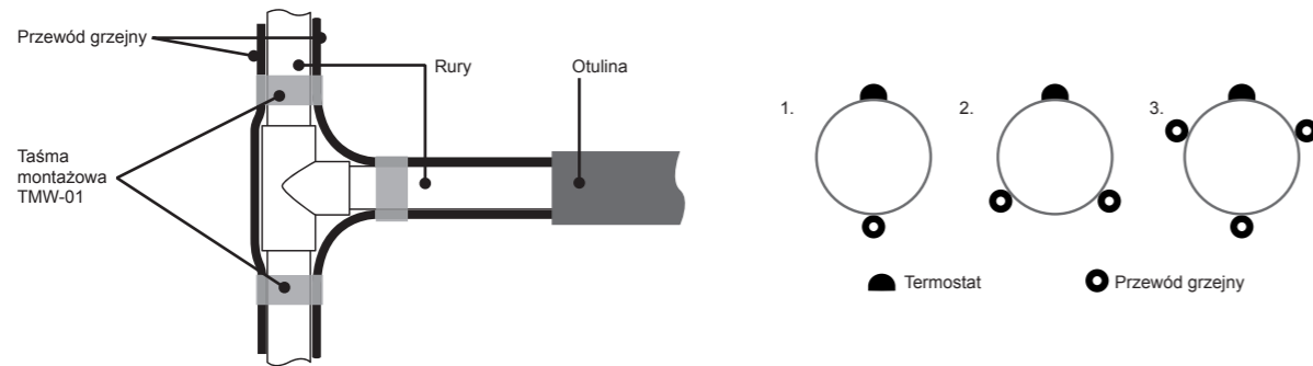
Rys. Wzdłużne ułożenie termostatu i przewodu grzejnego
